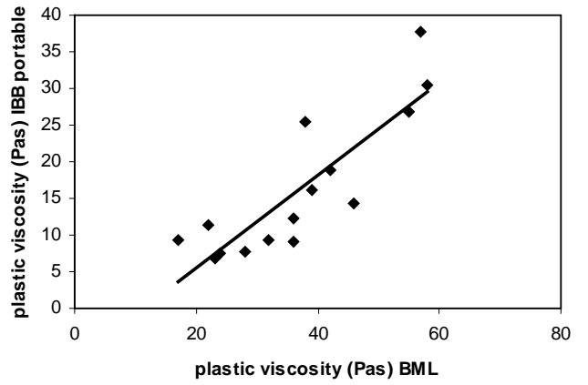
(d) plastic viscosity - IBB portable vs BML
