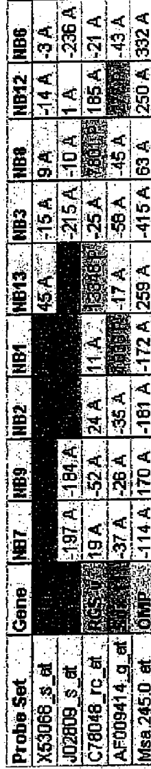
Microarray
